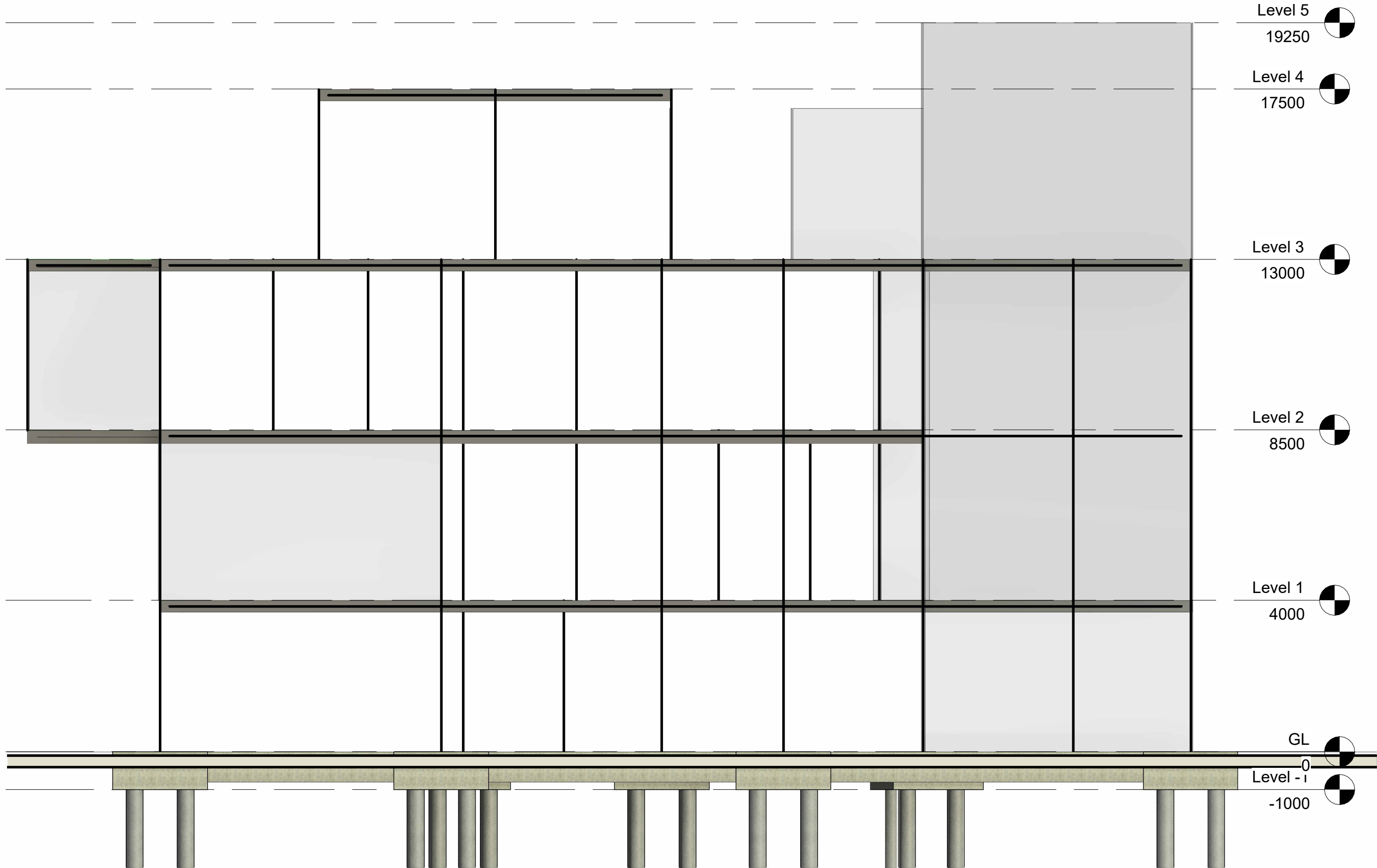
3 South 1 : 100
