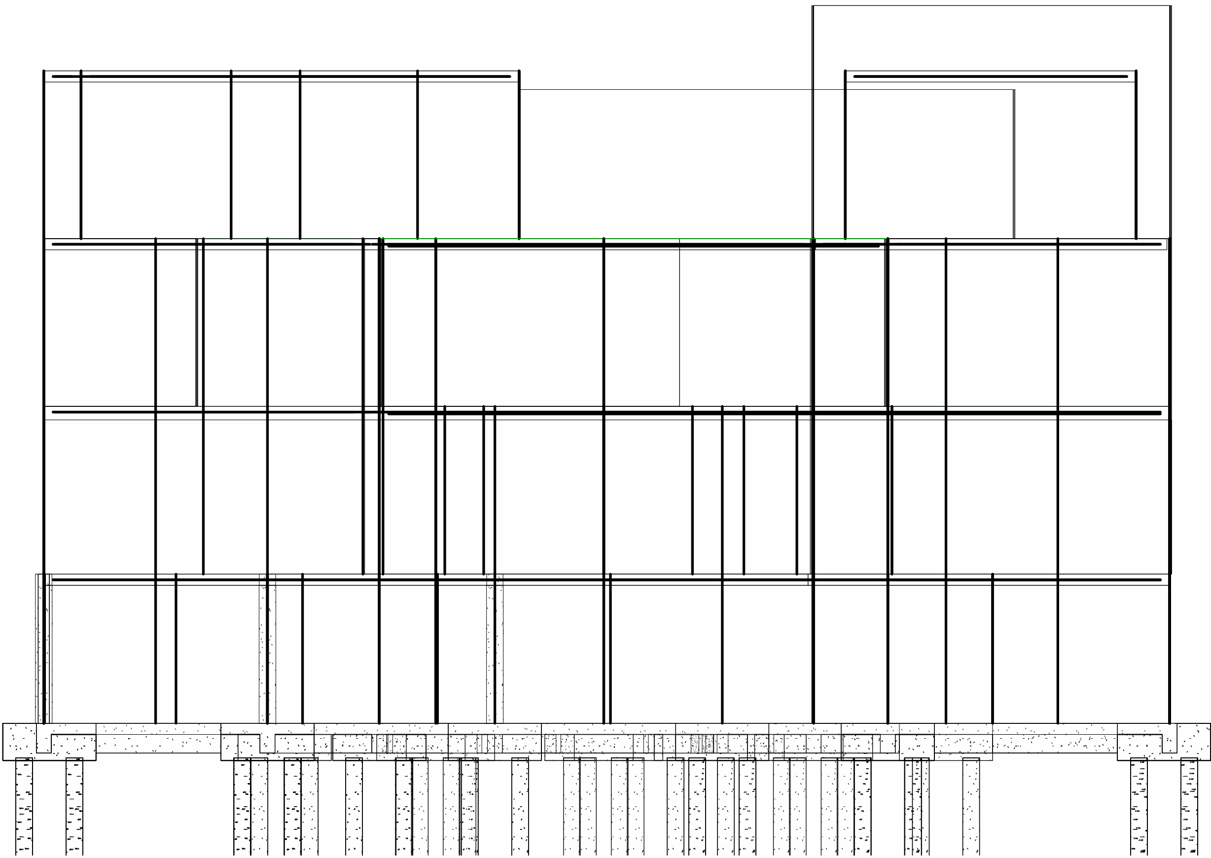
4 West 1 : 100
