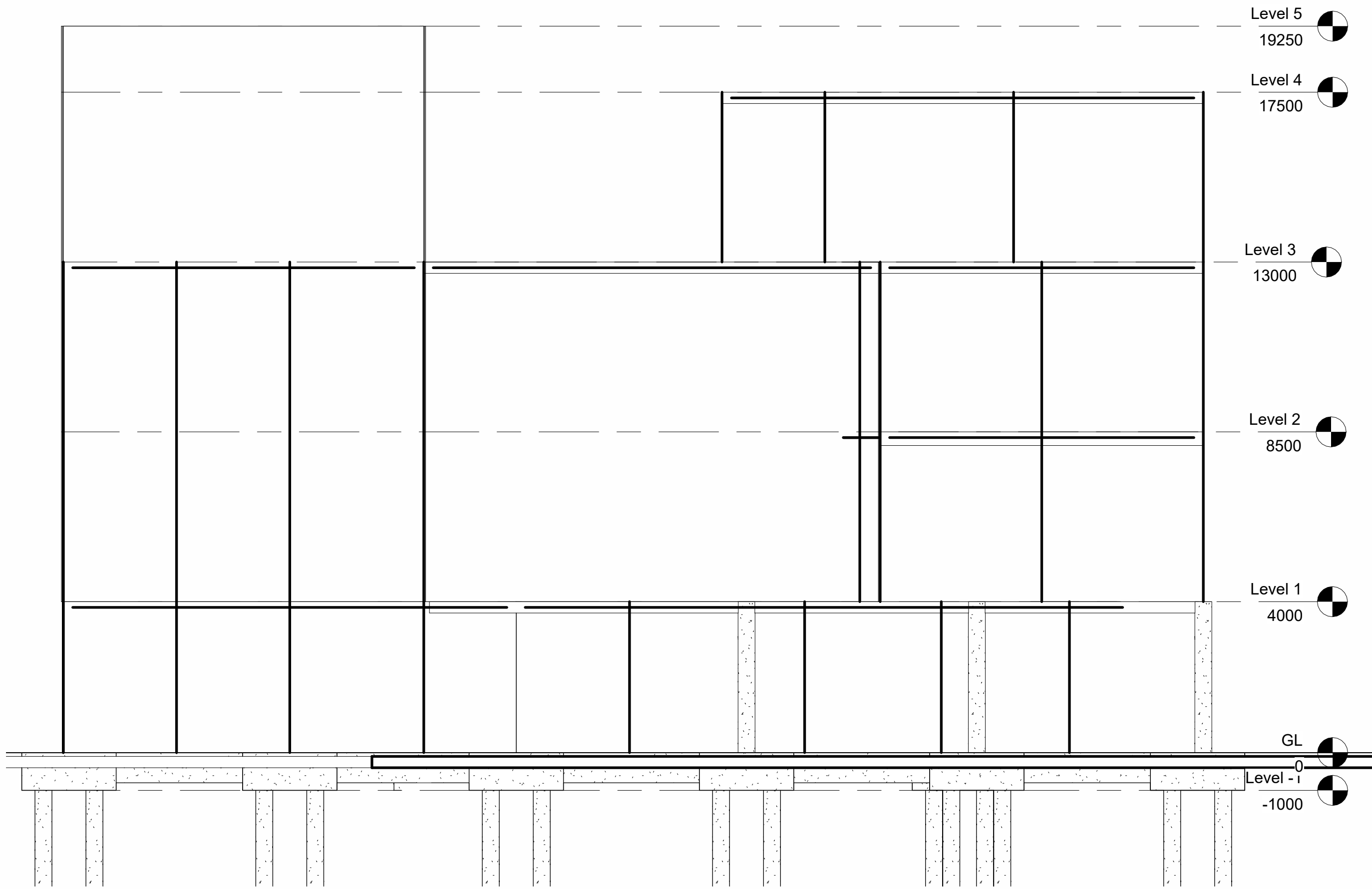
2 East 1 : 100
