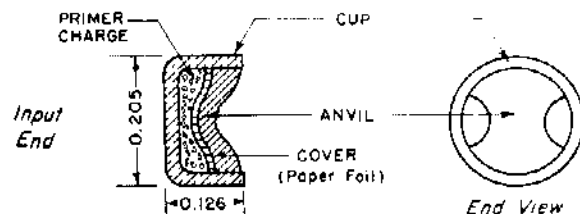
PERCUSSION PRIMER (M29A1)
