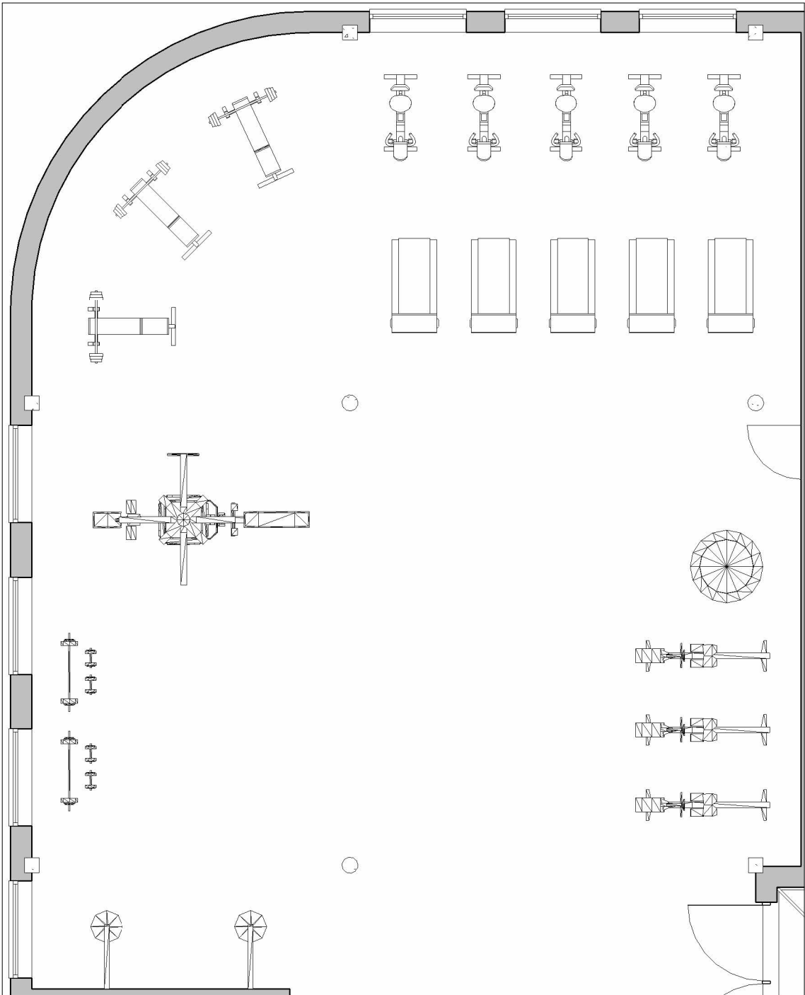
Gym 1 : 100
