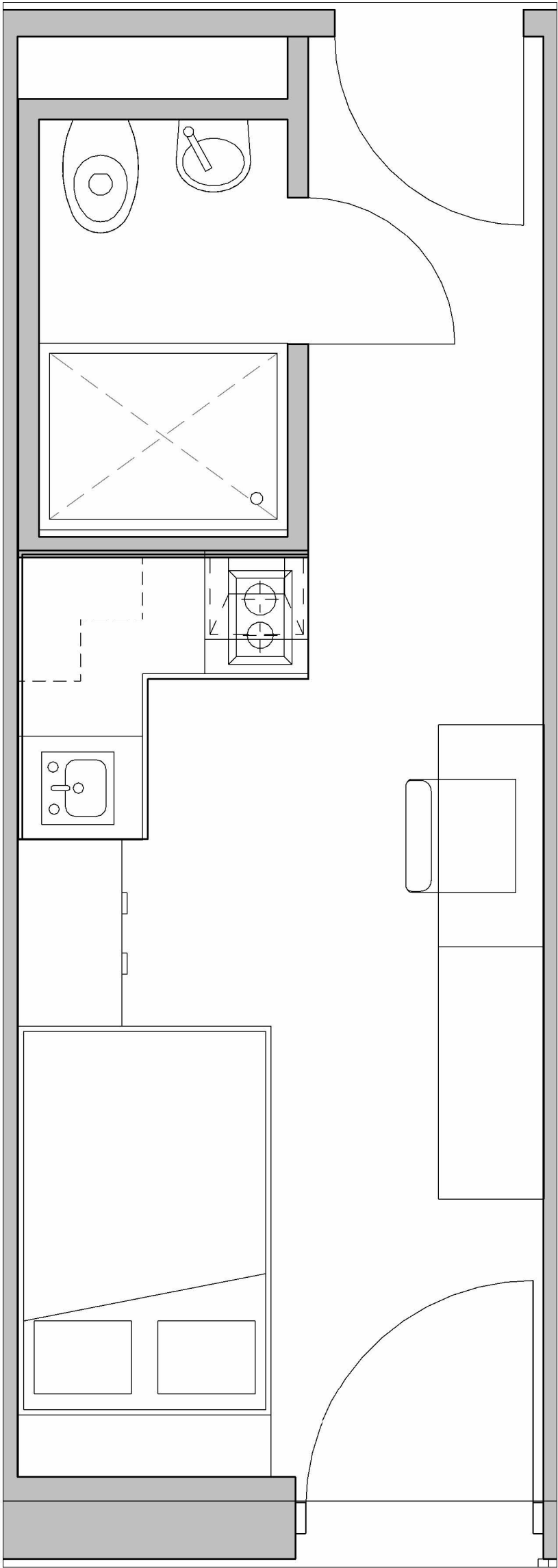
Studio Plan 1 : 25
