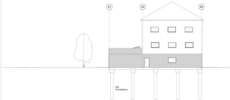
2 East 1 : 100
