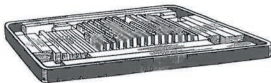
Fig. 18. Bulged Forme.
