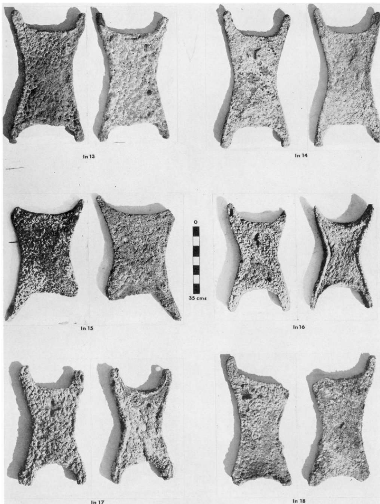
FIG. 58. Ingots In 13-In 18.
