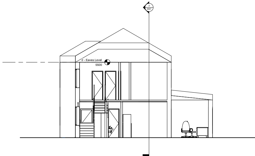
1 Section 1 1 : 50
