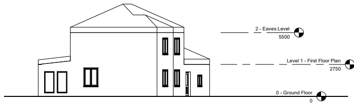
1 East 1 : 100
