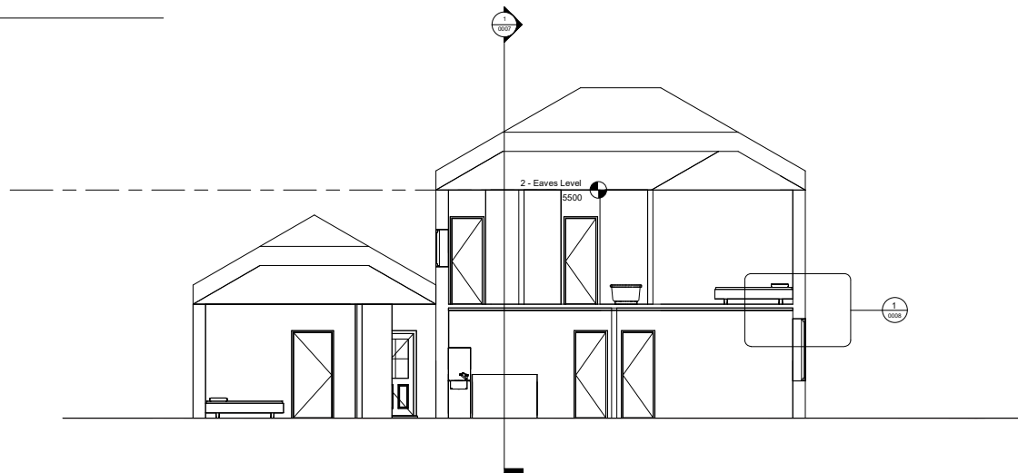
2 Section 2 1 : 50
