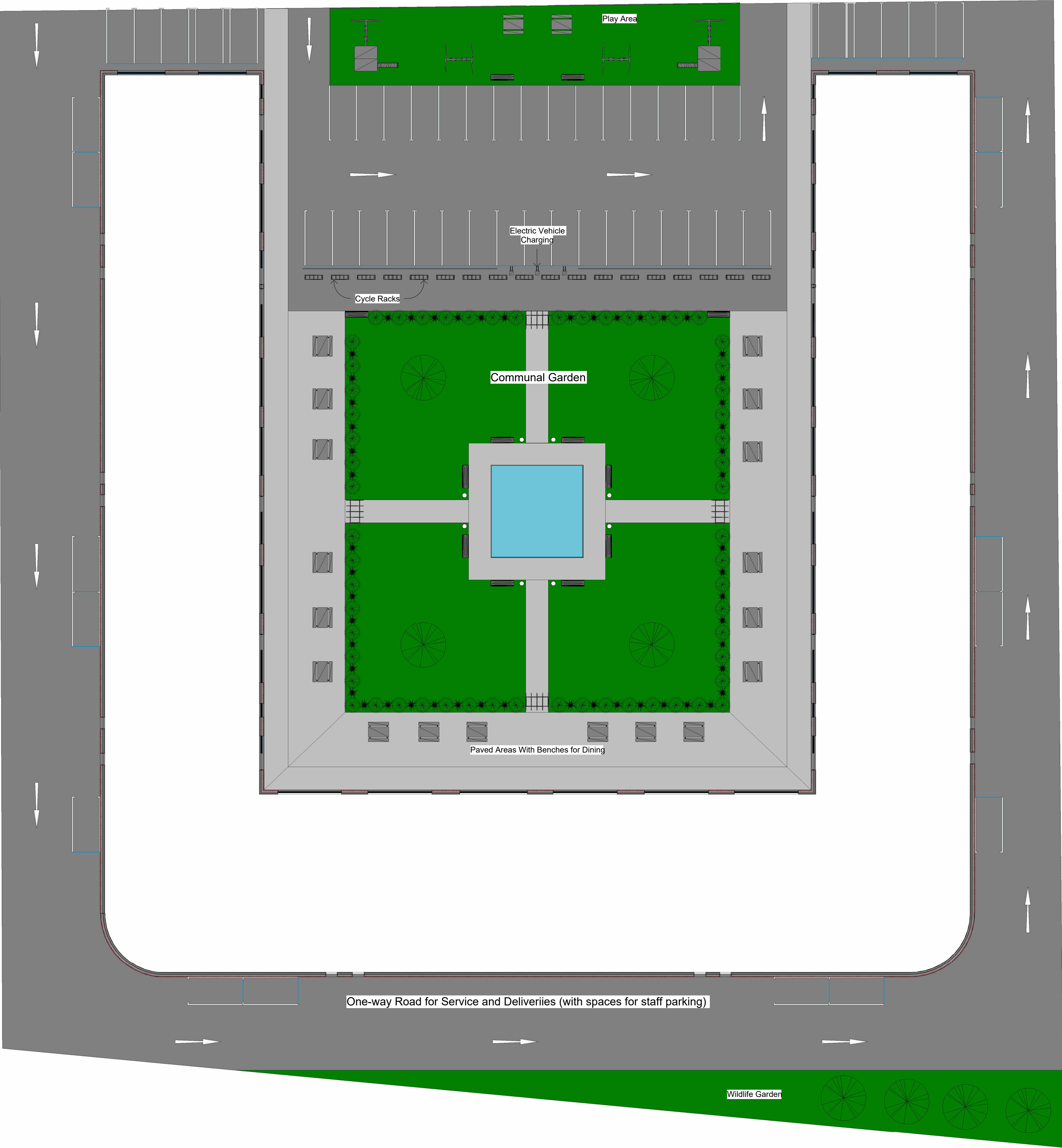
Site GA Plan 1 : 200
