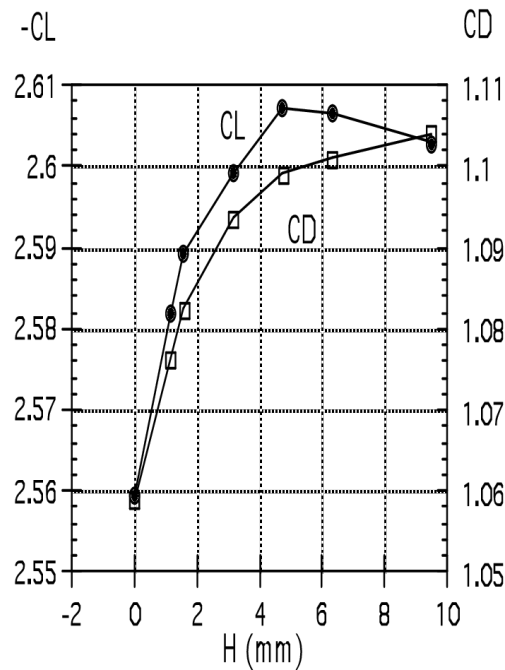
Figure 51 - Height vs -CL & Cd (Katz, 1995)
