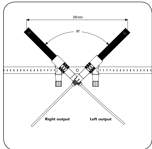
Fig. 26: NOS setup
