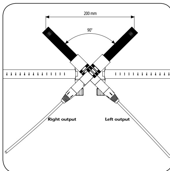
Fig. 24: DIN setup
