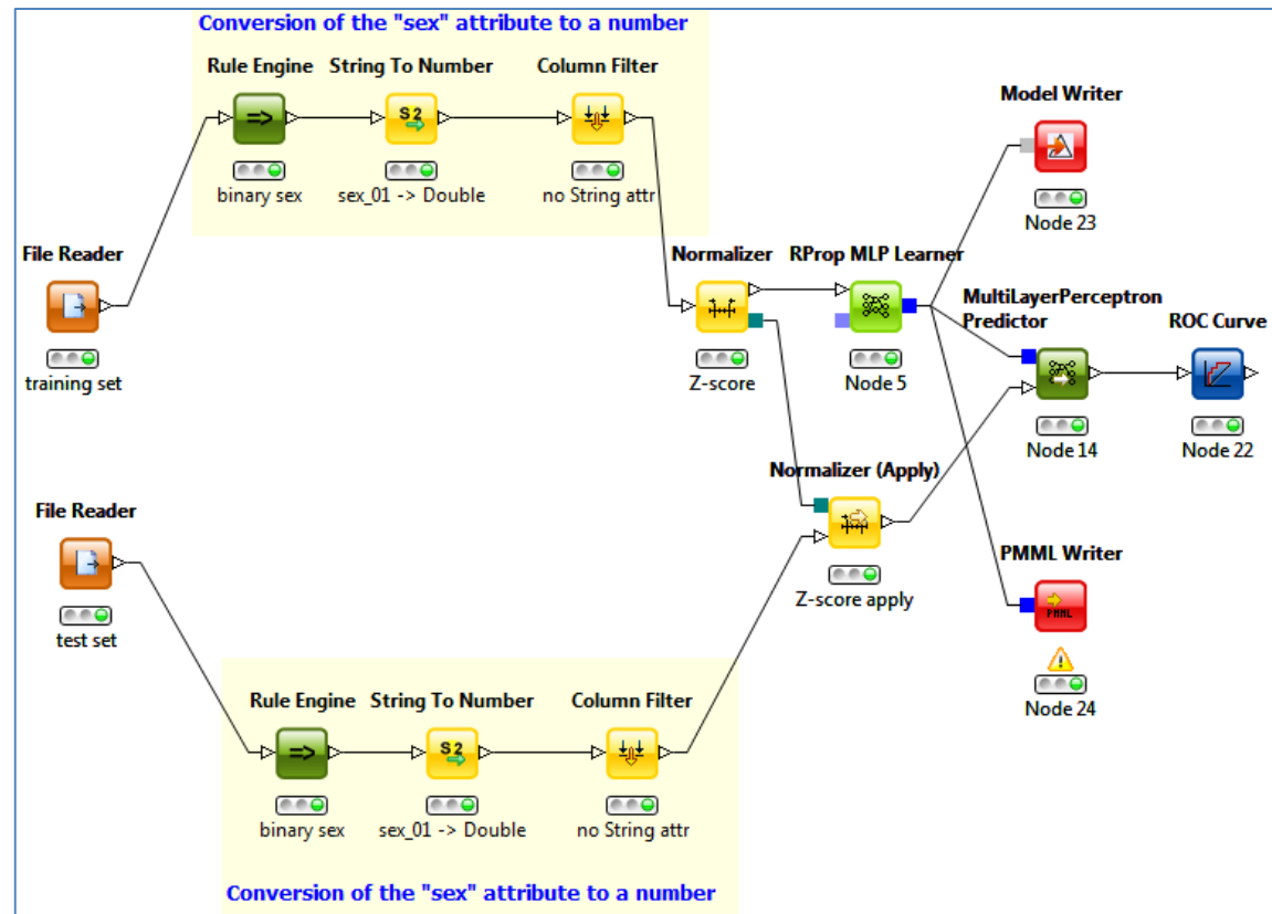
4.38. Workflow „my_first_ANN“
