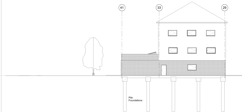
2 East 1 : 100
