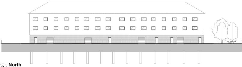
2 North 1 : 200
