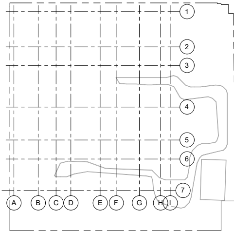
Existing site plan 1 : 300
