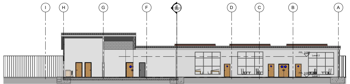
Section 1 1 : 100
