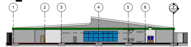
Section 2 1 : 200
