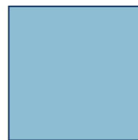
sgwâr
