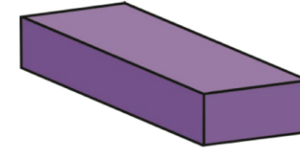
ciwboid
