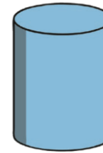
silindr
