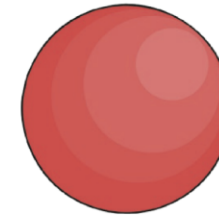
sffêr
