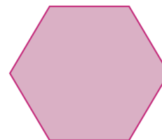
hecsagon
