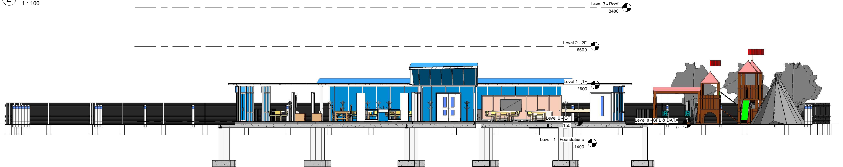
3 North 1 : 75
