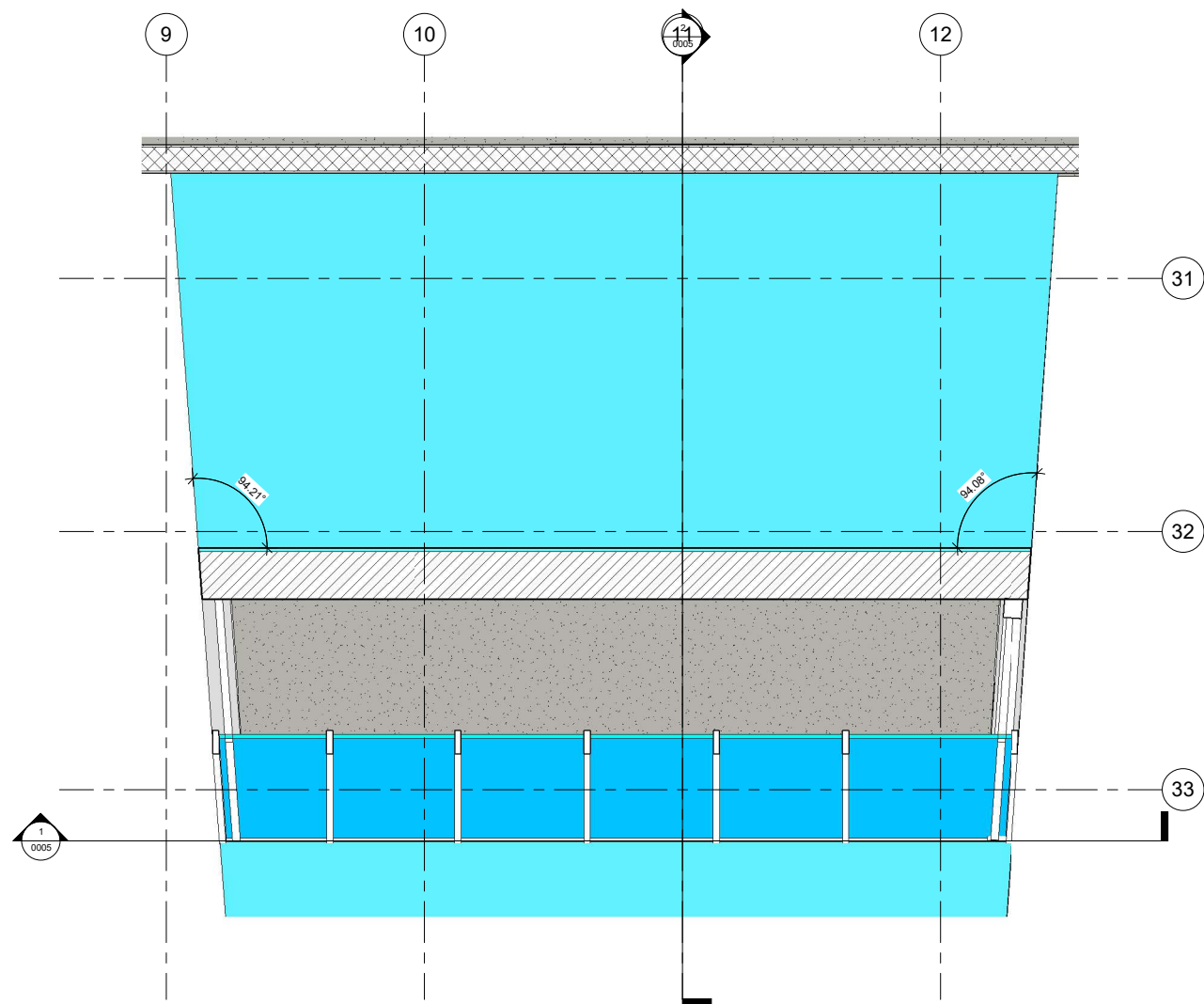
1 Detail 1 1 : 25
