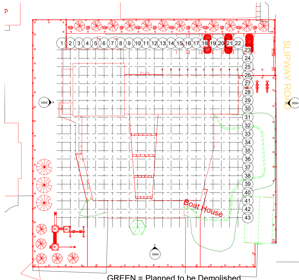
1 Site Works Plan 1 : 200
