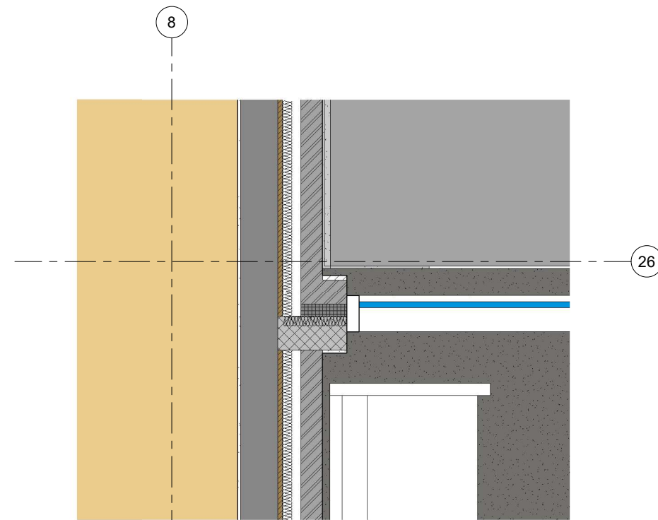
2 Detail 2 1 : 10
