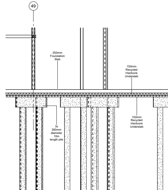
3 Section 1 - Callout 2 1 : 50
