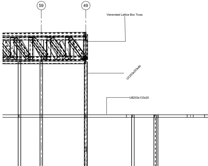
2 Section 1 - Callout 1 1 : 50
