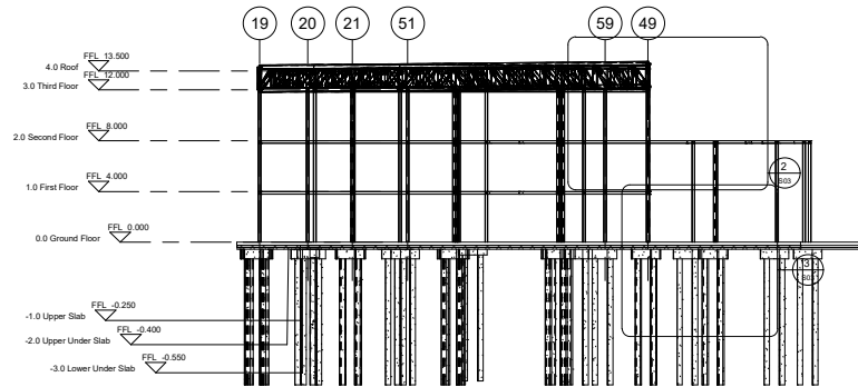
1 Section 1 1 : 200
