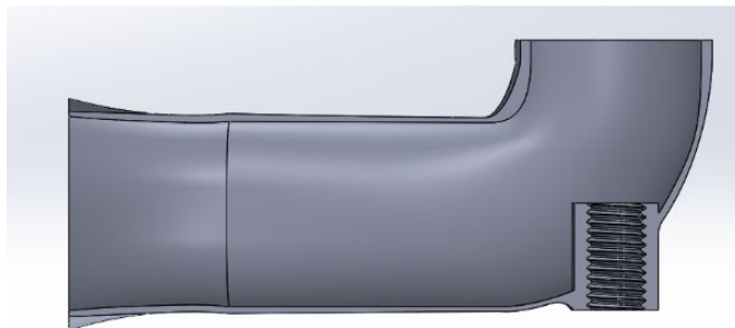
FIGURE 116: PORT 1 MINI PORT
