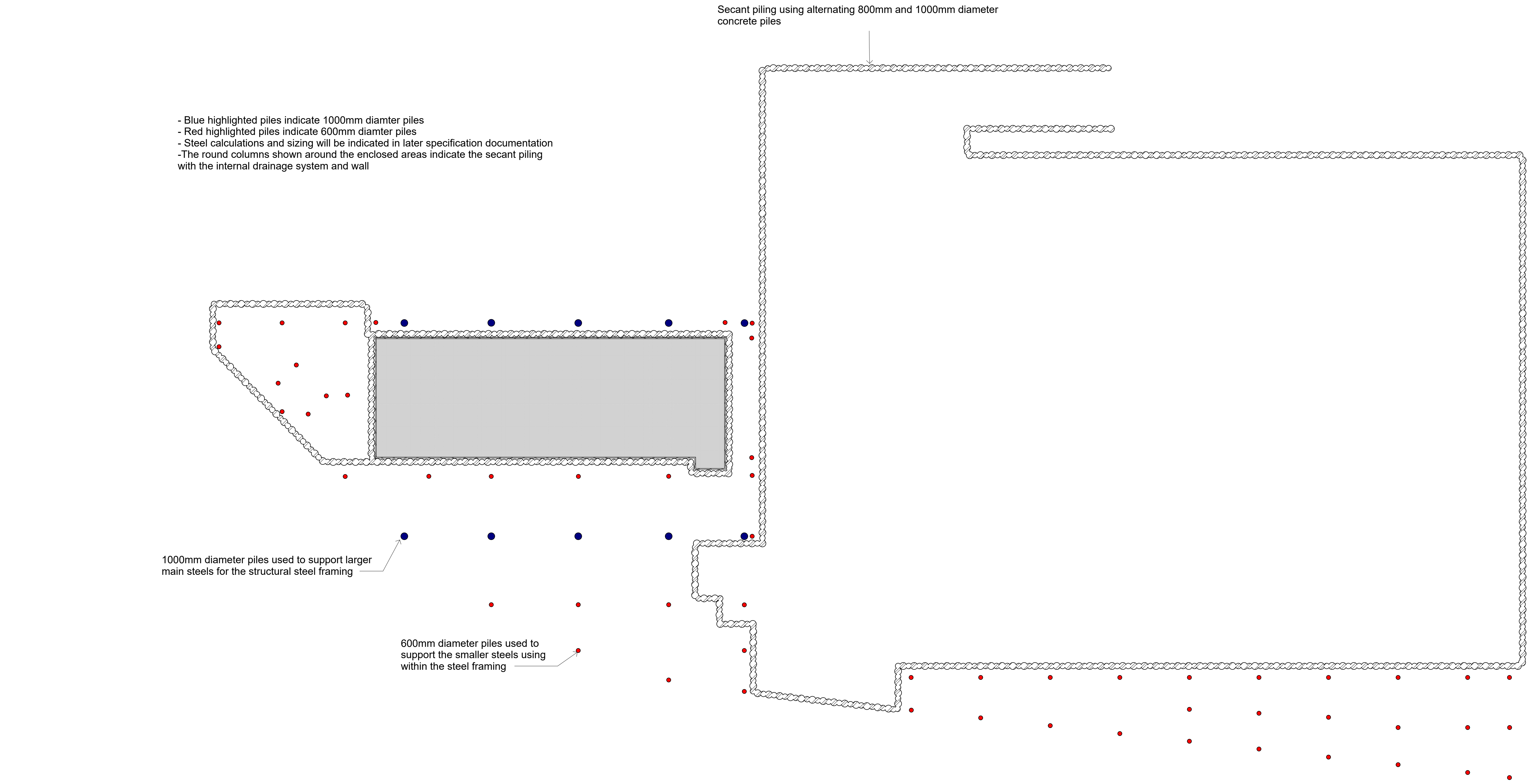
Piling Layout 1 : 300
