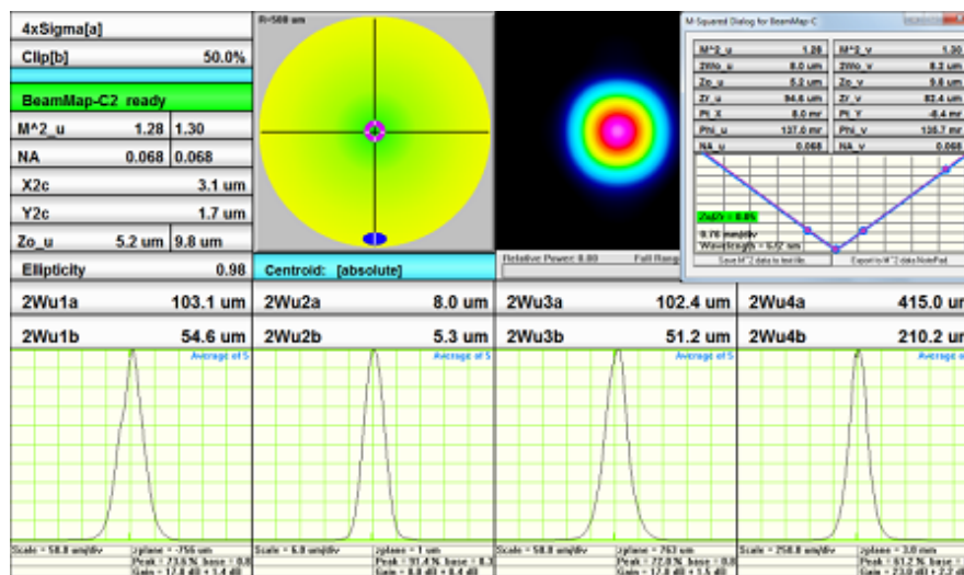
Figure 20 Using BeamMap2 Software
